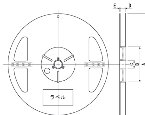
リール寸法
