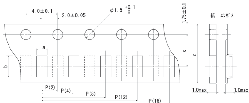
テープ寸法
